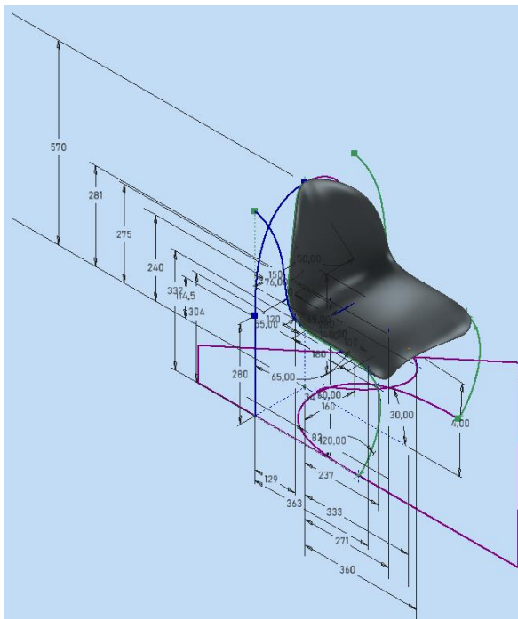
Obr. č. 19 - stolička s kótami
